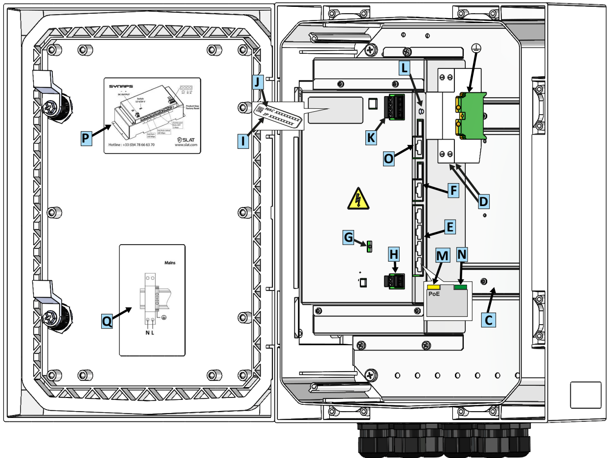
Figure 6-3 - Vue de l'intérieur du coffret
