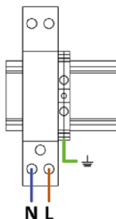
Figure 8-4 - Raccordement secteur
