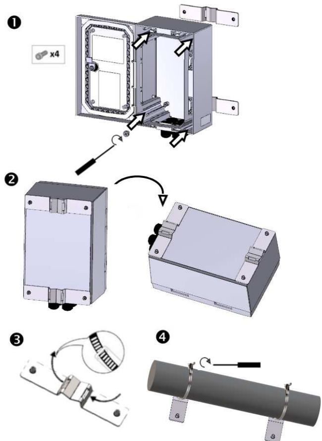
Figure 8-1 - Montage sur un mât/poteau
