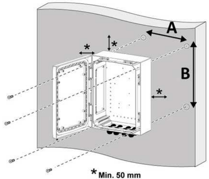
Figure 8-2 - Montage sur mur ou une chambre de tirage
