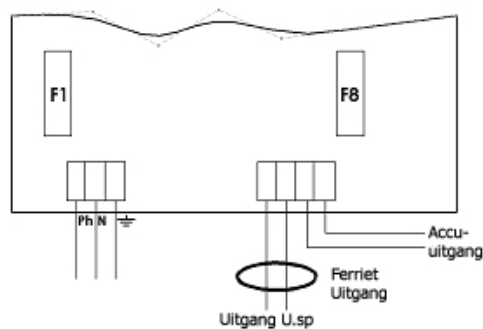
Kabels 100-150W
