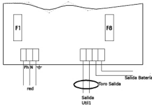
Cableado 100-150 W
