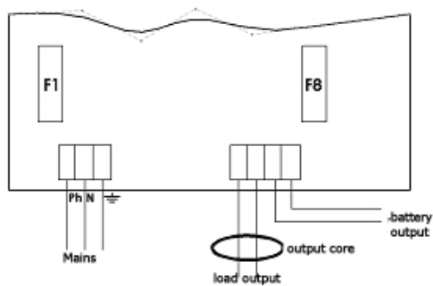
100-150 W wiring
