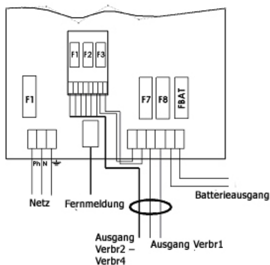
Platine mit 3 Sicherungsausgängen 100-150 W
