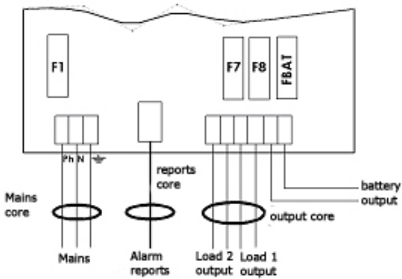
400-600 W wiring
