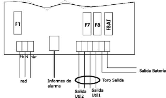
Cableado 100-300 W
